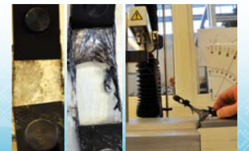
Fig. 4: Måling av strekkstyrke
